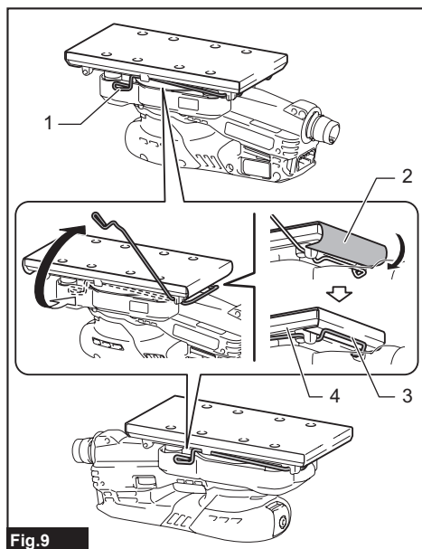
► 1. Palanca de sujeción 2. Papel abrasivo 3. Sujeción 4. Base
