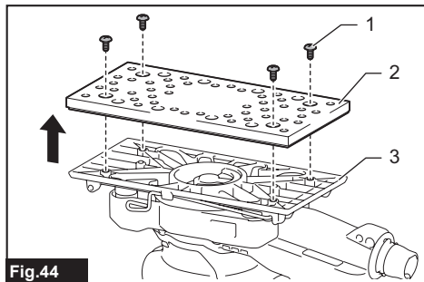
► 1. Vis 2. Patin 3. Socle
