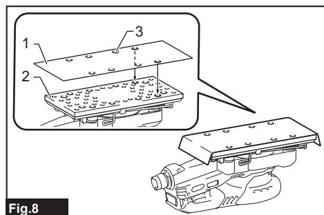
► 1. Papel abrasivo 2. Almohadilla 3. Orificio para succión de polvo
