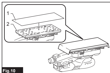
► 1. Papel abrasivo 2. Almohadilla
